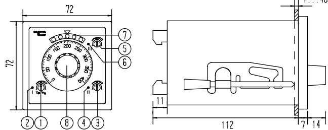
Schalttafelabschnitt 67,0x67,0mm
