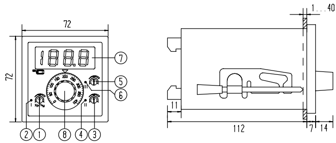
Schalttafelabschnitt 67,0x67,0mm
