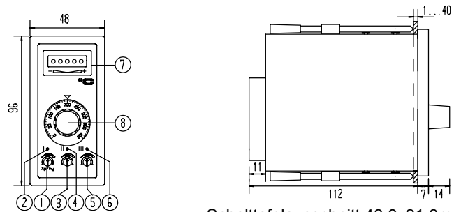
Schalttafelabschnitt 43,0x91,0mm
