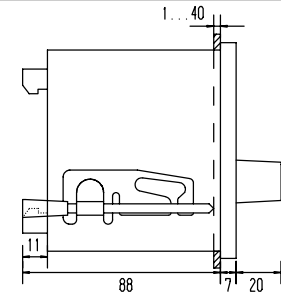
Schalttafel Ausschnitt 91,0x91,0mm
